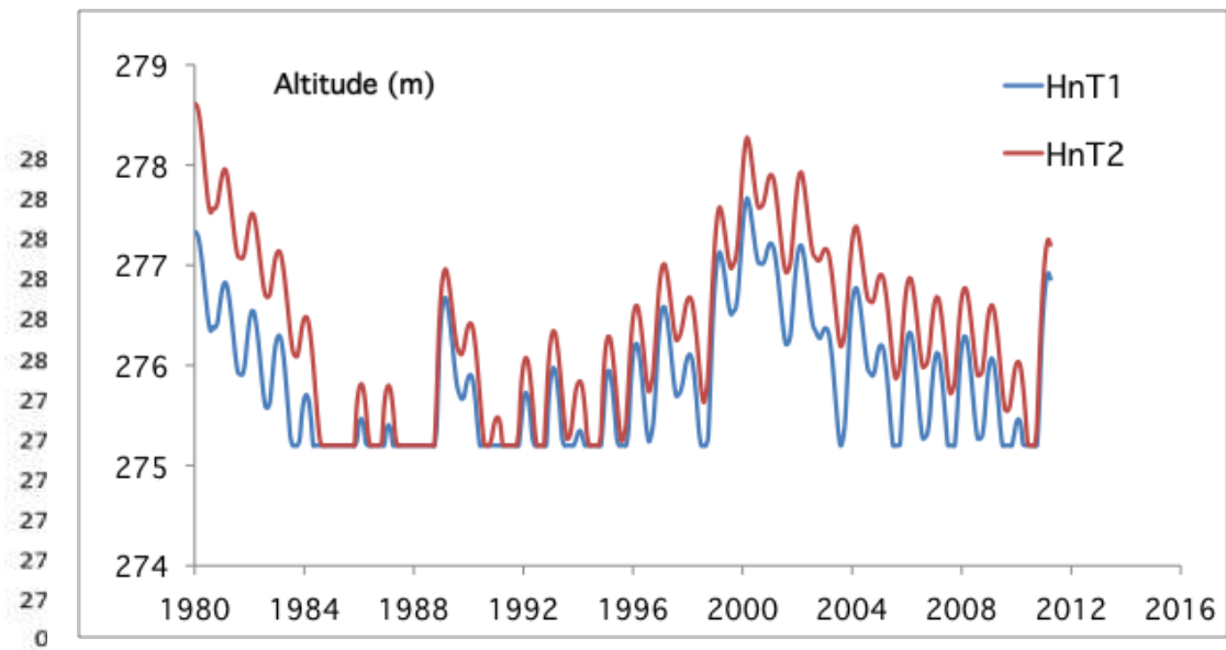
Figure 16 – Le niveau naturel reconstitué (en bleu, scénario HnT1) et le niveau simulé de la cuvette nord du Lac avec un apport supplémentaire de 3,4 \text{ km}^3/\text{an} (en rouge, scénario HnT2).
