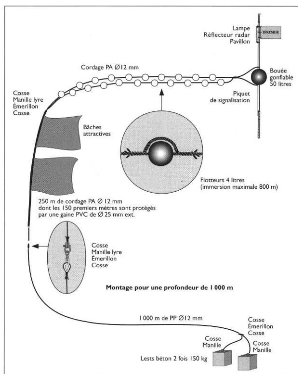
Fig. 11 Plan d'un DCP utilisé en Martinique.
