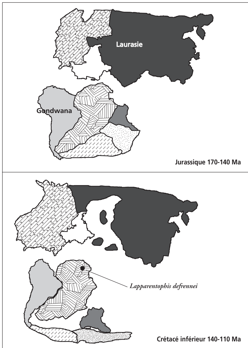
Figure 2 Localisation et datation des principaux fossiles d'Ophidiens
