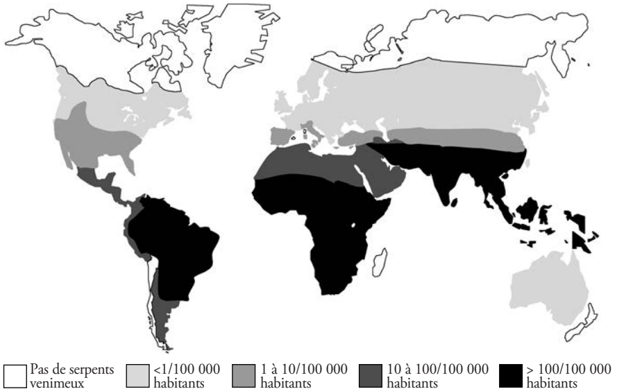
Figure 43 Distribution mondiale de la morbidité ophidienne
