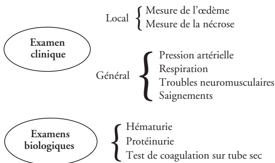
Figure 54 Principes de la surveillance clinique des envenimations opidiennes
