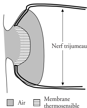
Figure 6 Schéma de la fossette thermosensible d'un crotale (d'après NEWMAN et HARTLINE, 1982)
