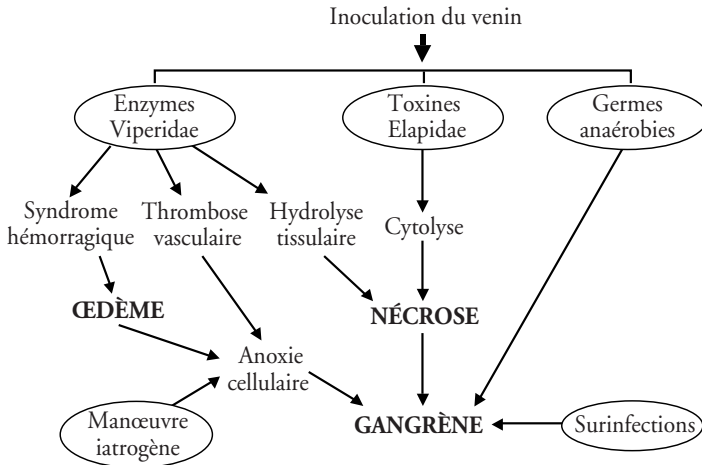
Figure 24 Étiopathogénie de la nécrose
