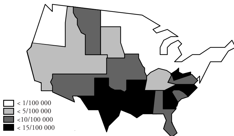
Figure 45 Morbidité ophidienne aux États-Unis (d'après PARRISH, 1980)
