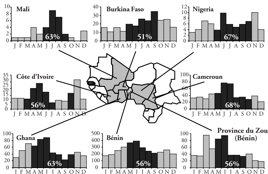
Figure 40 Variation saisonnière des morsures de serpent en Afrique de l'Ouest
