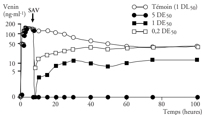
Figure 34 Effet de différentes doses de F(ab') 2 (d'après RIVIÈRE et al. , 1997)
