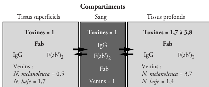
Figure 27 Diffusion du venin et de l'antivenin dans les compartiments biologiques (d'après ISMAIL et al. , 1996)
