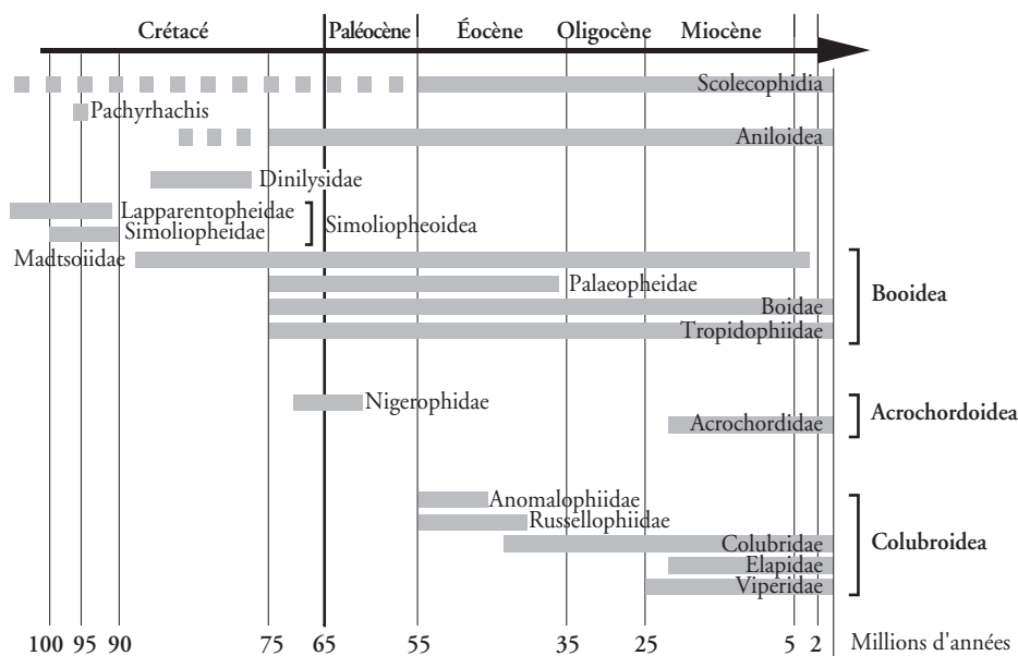
Figure 1 Datation stratigraphique des principales familles d'Ophidiens (d'après RAGE, 1982)
