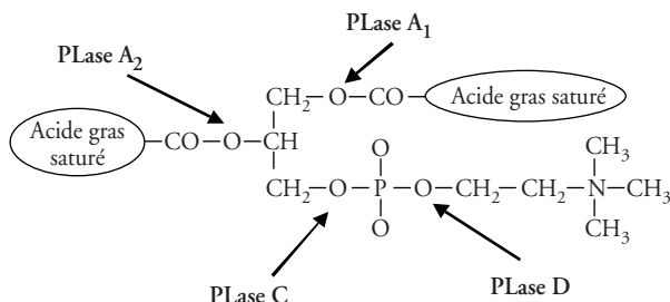
Figure 10 Site d'action des phospholipases
