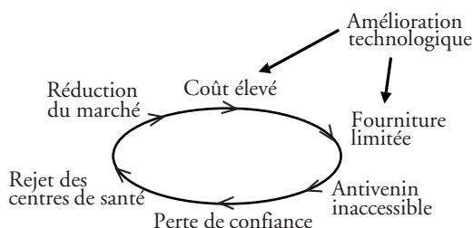
Figure 55 Cercle vicieux alimentant la mauvaise disponibilité des antivenins
