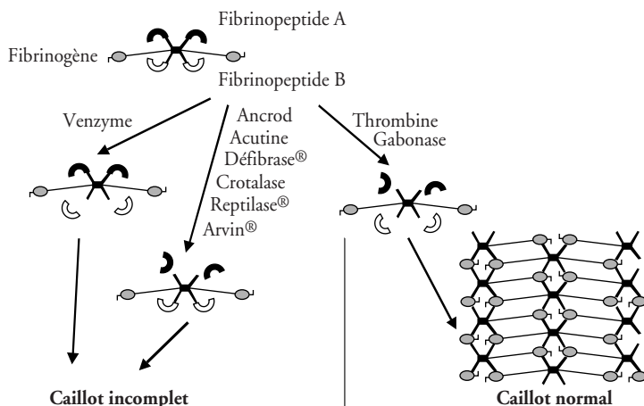
Figure 23 Intervention des venins de serpent sur la formation du réseau de fibrine
