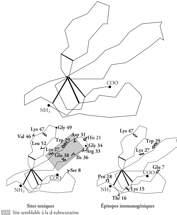
Figure 14 Structure moléculaire d'une neurotoxine- \alpha
