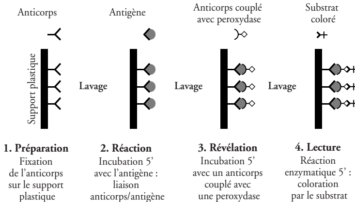
Figure 31 Mécanisme du test Elisa
