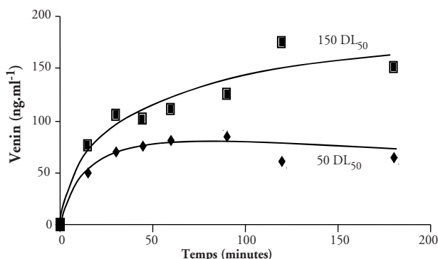
Figure 26 Diffusion du venin dans le secteur vasculaire après administration par voie intramusculaire (d'après AUDEBERT et al. , 1994)
