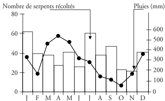
Figure 38 Variation saisonnière de l'abondance des serpents en Guyane française
