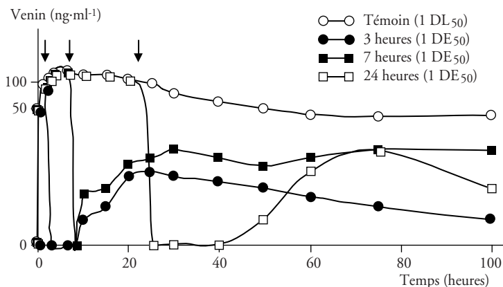
Figure 33 Effet du délai d'administration des F(ab')_2 (d'après RIVIÈRE et al. , 1997)
