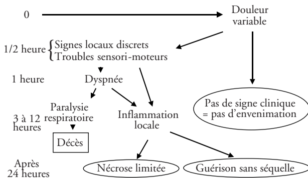
Figure 47 Chronologie d'une envenimation par Elapidae
