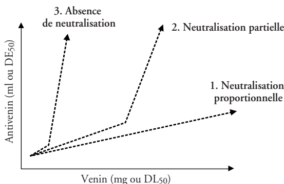
Figure 30 Courbes théoriques de neutralisation
