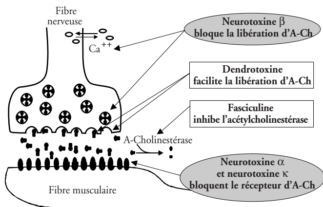
Figure 17 Mode d'action des neurotoxines de serpent
