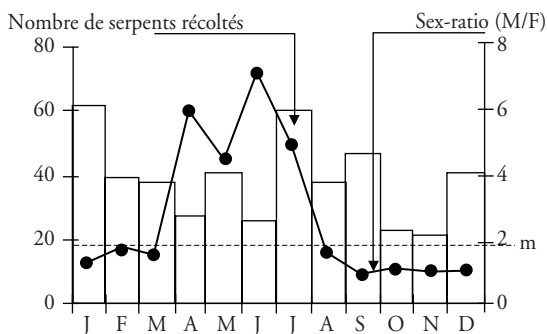
Figure 37 Variation saisonnière du sex-ratio des serpents en région équatoriale humide (Guyane française)
