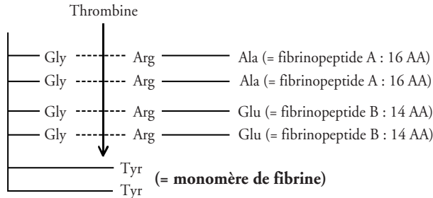
Figure 20 Transformation du fibrinogène en monomère de fibrine (d'après SAMAMA, 1990)
