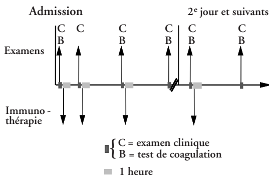
Figure 53 Protocole d'immunothérapie
