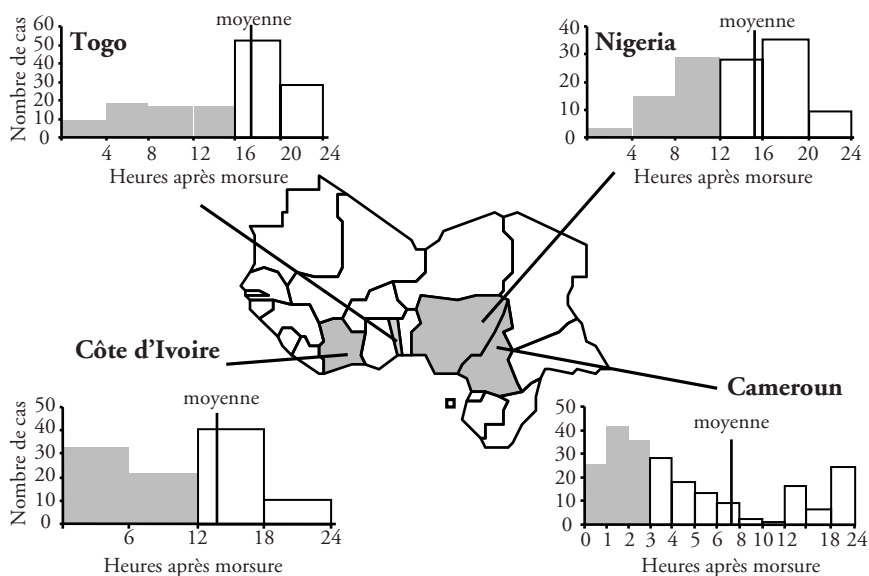
Figure 46 Délais de consultation après morsure de serpent en Afrique de l'Ouest
