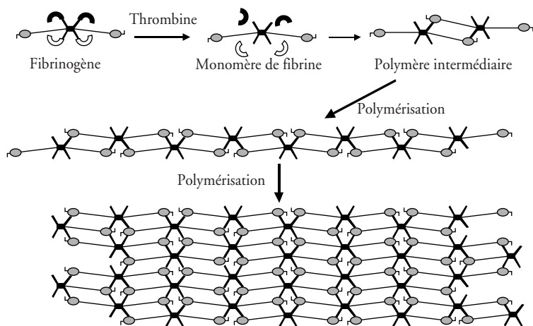
Figure 21 Formation du réseau de fibrine (d'après SAMAMA, 1990)
