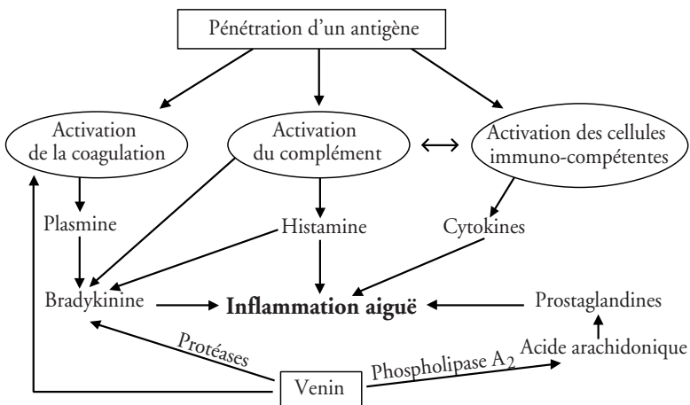
Figure 25 Mécanismes de l'inflammation
