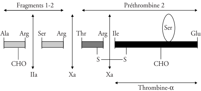
Figure 19 Sites d'hydrolyse de la molécule de prothrombine (d'après SAMAMA, 1990)
