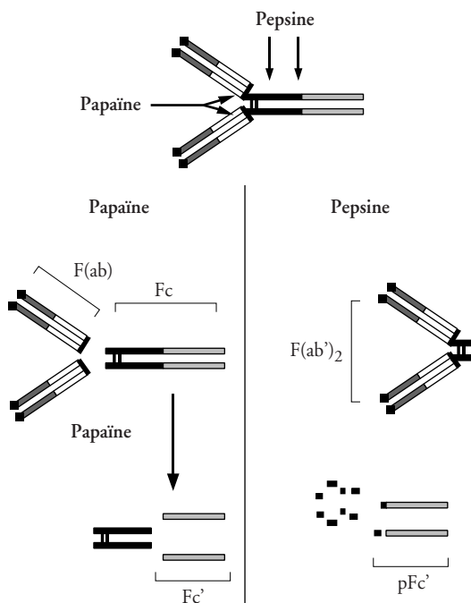
Figure 29 Fractionnement des immunoglobulines thérapeutiques
