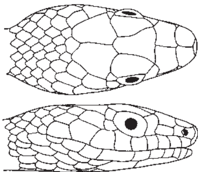
Figure 7 Écaillure de la tête d'un colubridae
