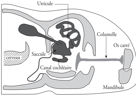
Figure 4 Schéma de l'oreille interne des serpents
