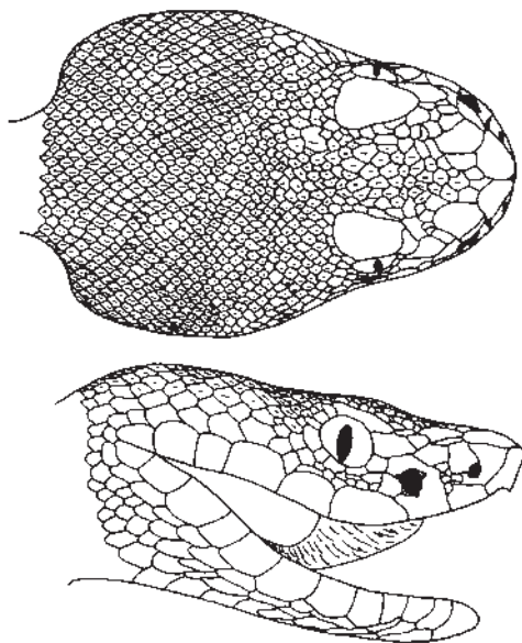
Figure 8 Écaillure de la tête d'un viperidae
