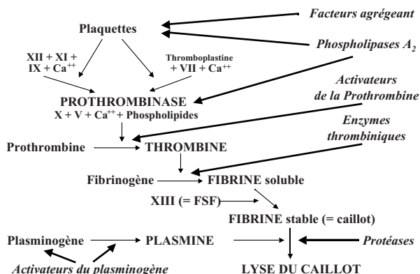
Figure 22 Intervention des venins de serpent sur la coagulation sanguine
