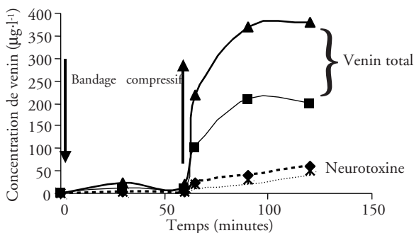
Figure 51 Effet d'un bandage compressif sur la diffusion du venin
