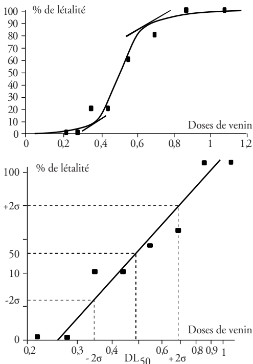
Figure 15 Détermination graphique de la toxicité moyenne ( DL_{50} )
