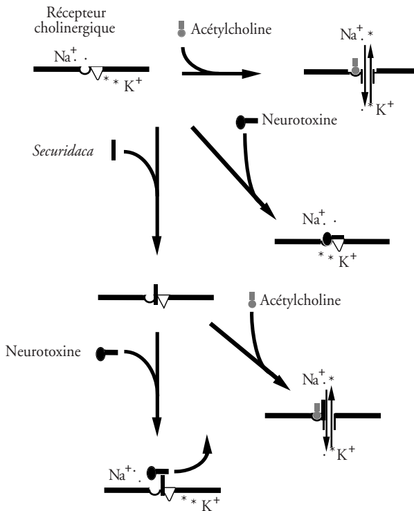
Figure 28 Mode d'action de Securidaca
