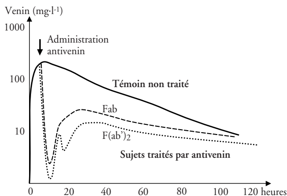
Figure 32 Neutralisation du venin par les fragments d'immunoglobulines (d'après RIVIÈRE ET BON, 1999)
