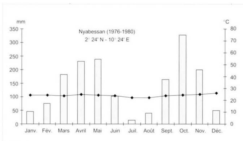
Fig. 5 – Diagramme ombrothermique des précipitations moyennes (en mm) et des températures mesurées à Nyabessan
