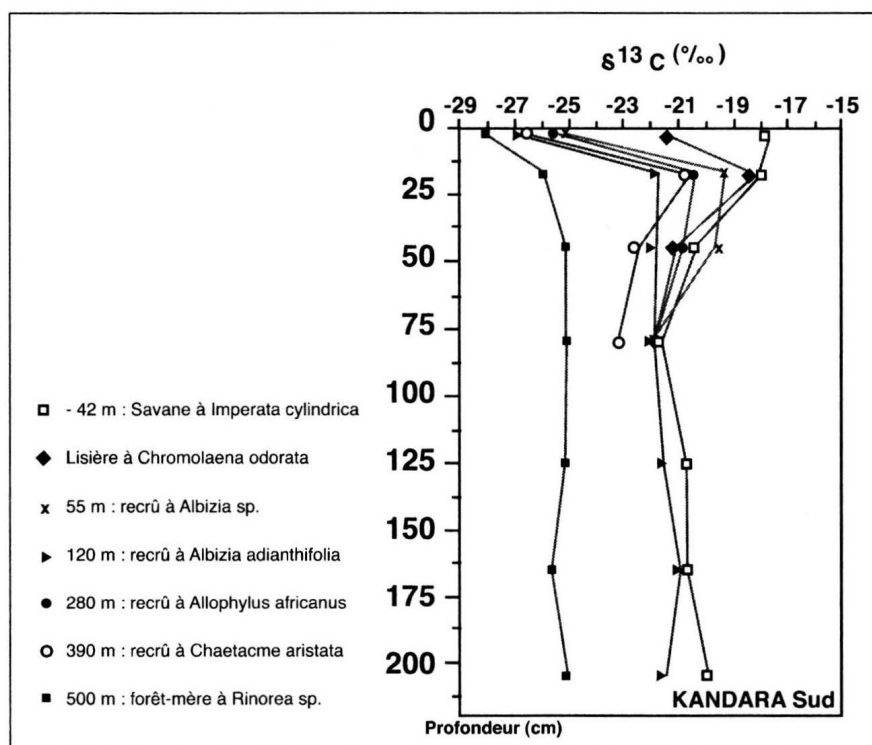
Figure 1. Variation de la composition isotopique dans le sol de la savane, de la forêt mère, et dans les recrûs forestiers qui vont de la lisière à la forêt-mère.
