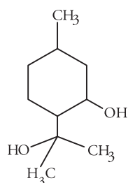
p -menthane-3,8-diol(PMD extrait d' Eucalyptus maculata citriodora )
