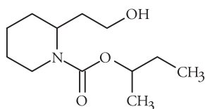
[1-pipéridine acide carboxylique, 2(2-hydroxyéthyl)-, 1-méthylpropylester] (KBR3023 ou picaridine)
