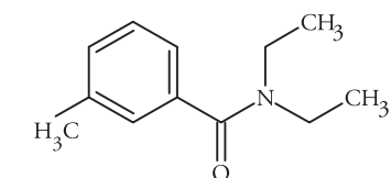
N,N -diéthyl- m -toluamide (DEET)
