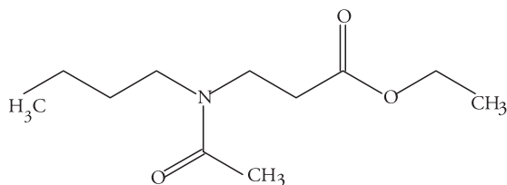
[3-( N -acétyl- N -butyl) acide aminopropionique éthyl ester] (Merck IR3535 ® )
