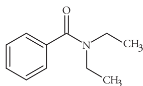
N,N -diéthyl phénylacétamide (DEPA)
