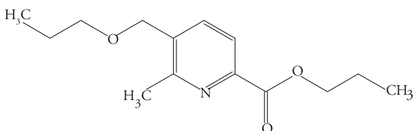
MGK 326 di- n -propyl-isocinchomérone
