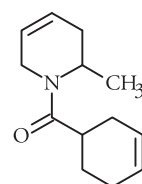
[1,-(3-cyclohexene-1-yl-carbonyl)-2-méthyl pipéridine] AI337220
