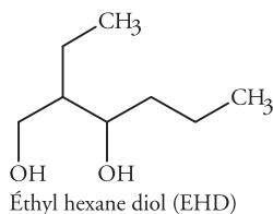
Éthyl hexane diol (EHD)
