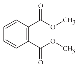
diméthyl phthalate (DMP)
