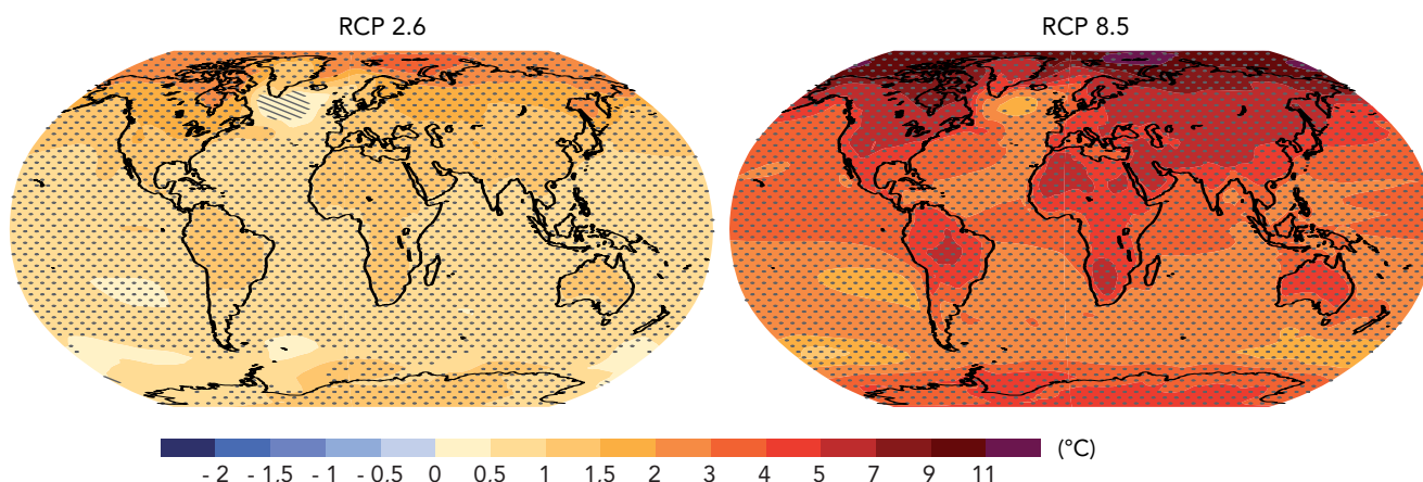
Figure 17. Évolution de la température moyenne en surface entre 1986-2005 et 2081-2100.
