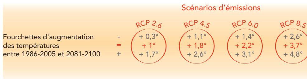
Figure 15. Les projections climatiques de température, entre 1986-2005 et 2081-2100, en fonction des 4 scénarios d'émissions du Giec. Source : Giec, 2013.
