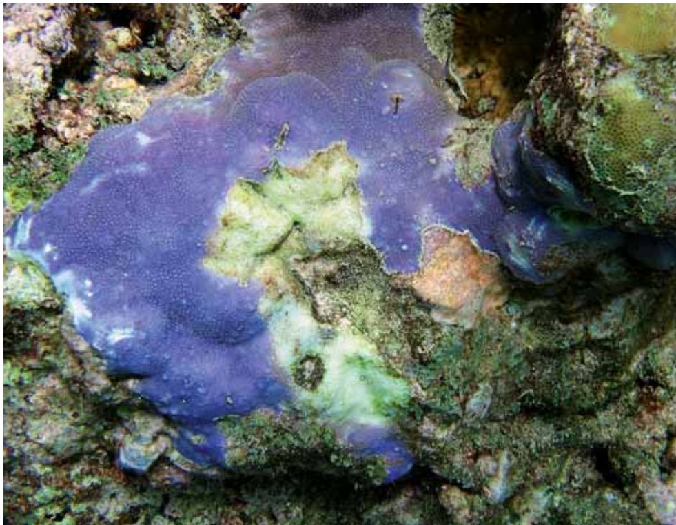
Maladie des taches blanches sur une colonie de porites à Mayotte.
