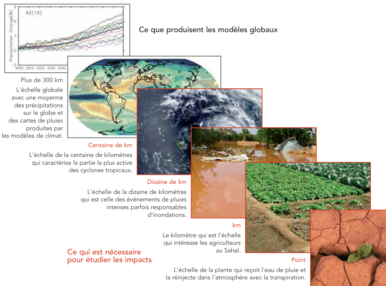
Figure 11. Illustration de la descente d'échelle dans le domaine du changement climatique et de ses impacts.
