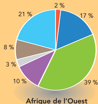
Figure 20. Répartition des sources d'émissions (monde, Afrique, Afrique de l'Ouest) en pourcentage.
