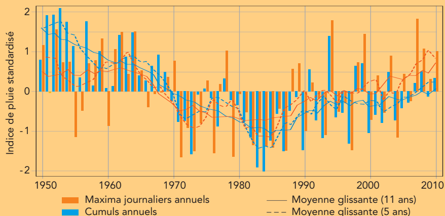
Figure 23. Évolution comparée des totaux et des maxima annuels de pluie sur le Sahel central (fenêtre 9,5° N-15,5° N 5° O-7° E) entre 1950 et 2010.
