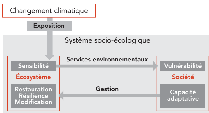
Figure 32. Exposition d'un système socio-écologique aux effets du changement climatique.
