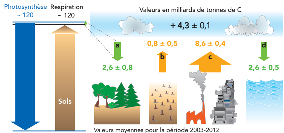
Figure 25. Échanges de carbone entre les écosystèmes et l'atmosphère. a/ Séquestration de carbone dans les sols, résultat de l'échange gazeux entre la photosynthèse et la respiration des plantes et des organismes et micro-organismes du sol. b/ Flux de carbone des sols vers l'atmosphère suite à la déforestation. c/ Émissions anthropiques de CO 2 non agricoles ou forestières. d/ Puits océanique. Sources : BERNOUX et CHEVALLIER, 2013 et www.globalcarbonproject.org
