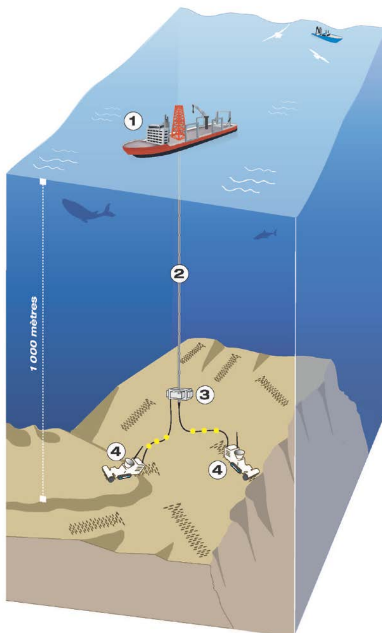
Figure 1 – Vision futuriste de ce que pourrait être une « mine sous-marine » en Polynésie française. Sur le schéma : 1/ structure de surface type navire minier : réception des matériaux et alimentation en énergie des engins de fond de mer, transport des matériaux vers un port ou une plateforme à proximité ; 2/ riser : liaison fond-surface, tube flexible de remontée des matériaux et câble pour l'énergie ; 3/ pompe : propulsion du matériau broyé dans le riser (air lift) ; 4/ engins miniers autopropulsés : extraction, fragmentation et ramassage des matériaux (croûtes polymétalliques). Source : ©IRD/ L. CORSINI
