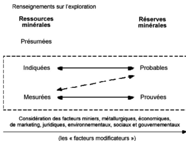
Figure 1 – Relations entre les ressources et les réserves minérales (source: CIM (2005))
