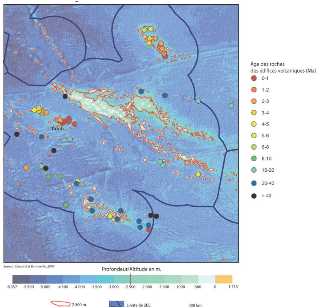
Figure 31 – Age des édifices volcaniques en Polynésie française (d'après Clouard et Bonneville, 2004)
