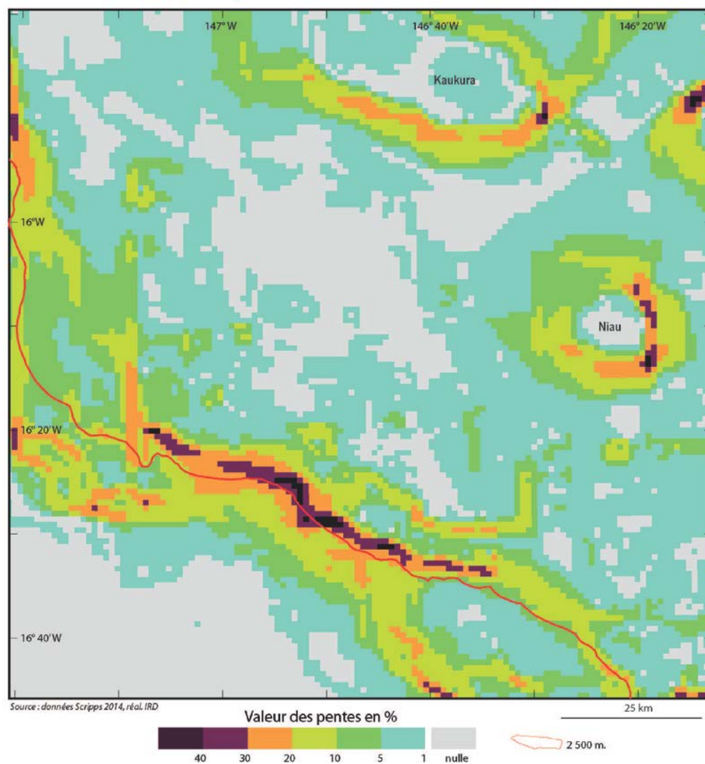
Figure 26 – Carte des pentes du secteur de Kaukura et Niau
