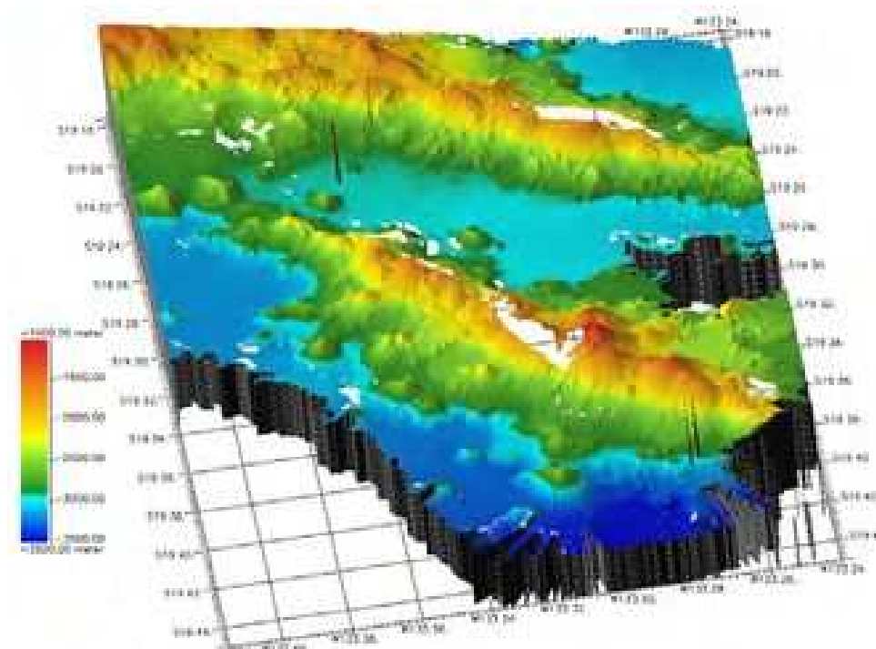
Figure 1 – Exemple de carte bathymétrique réalisée lors de la campagne Polyplac 2015. Les fonds sous-marins cartographiés pendant la campagne deux dragues ont été réalisés sur cet édifice ©Ifremer
