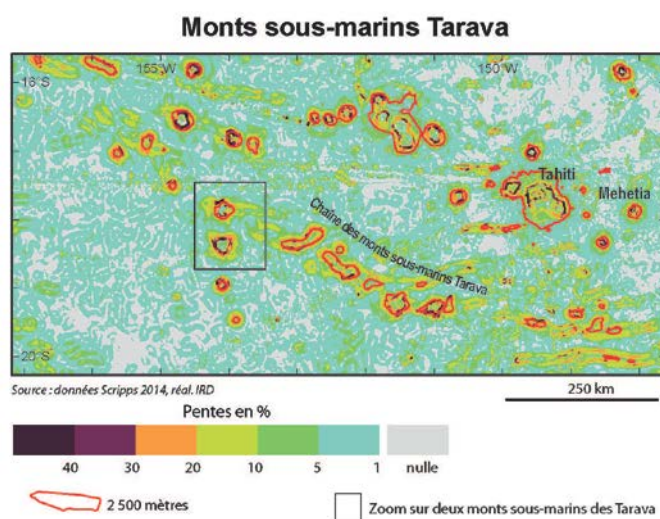
Figure 7 – Carte des pentes de la région des monts Tarava et îles de la Société
