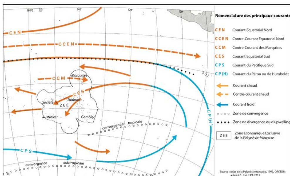
Carte 1 – Les courants marins dans le Pacifique centre Sud et le grand gyre du Pacifique Sud (Atlas de la Polynésie française, 1993, Orstom).
