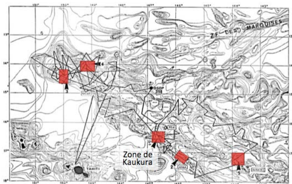
Figure 12 – Carte bathymétrique du plateau des Tuamotu, montrant les transects (trait épais) réalisés dans le programme Nodco ainsi que les zones qui ont été étudiées en détail (encadrés rouges) dans ce programme (Source : Bougault et Saget, 2012). NB : ces zones encadrées ne sont pas forcément les sites les plus intéressants. La zone de Kaukura, qui contient des indices de minéralisation, est détaillée dans la figure 13.
