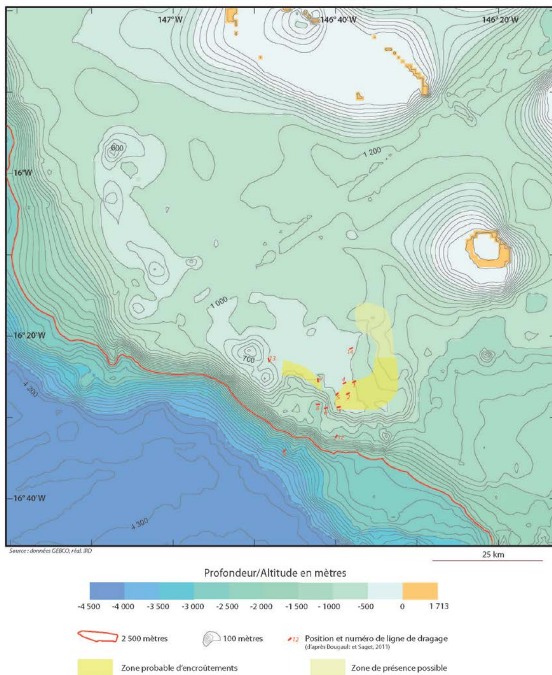
Figure 20 – Bathymétrie du secteur de Kaukura et Niau
