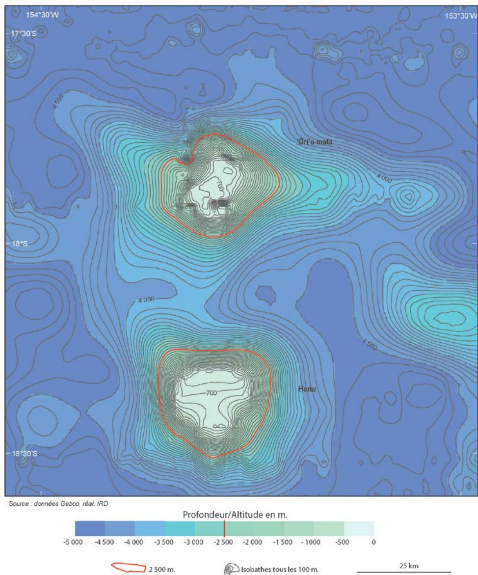
Figure 22 – Bathymétrie des monts sous-marins 'Ori'o mata et Honu (monts Tarava) (nommés par des élèves des collèges des îles sous le Vent, dans le cadre du programme Zepolyf)
