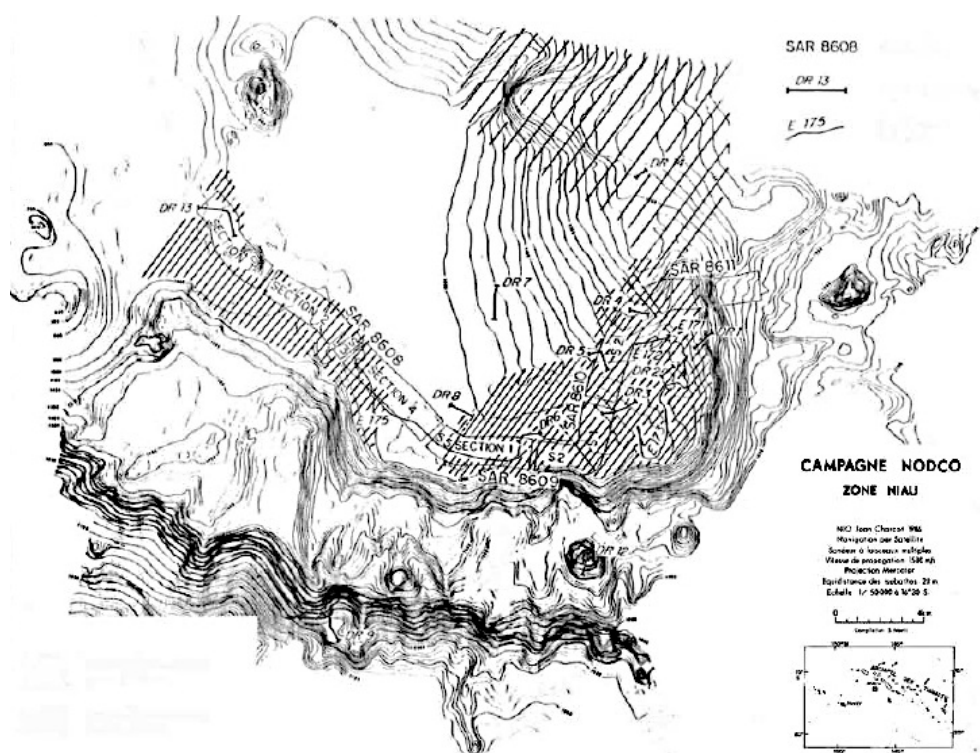
Figure 13 – Carte bathymétrique de la zone Kaukura du plateau de Tuamotu. Les « hachures serrées » représentent la zone d'encroûtements la plus favorable et les « hachurés larges » représentent la zone de présence possible d'encroûtements (Source : Bougault et Saget, 2012).
