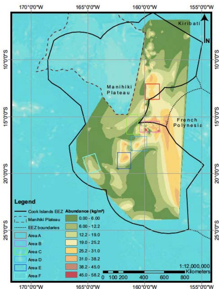
Figure 15 – Répartition des nodules polymétalliques dans les régions à l'ouest de la ZEE de Polynésie française (Hein et al. , 2015)
