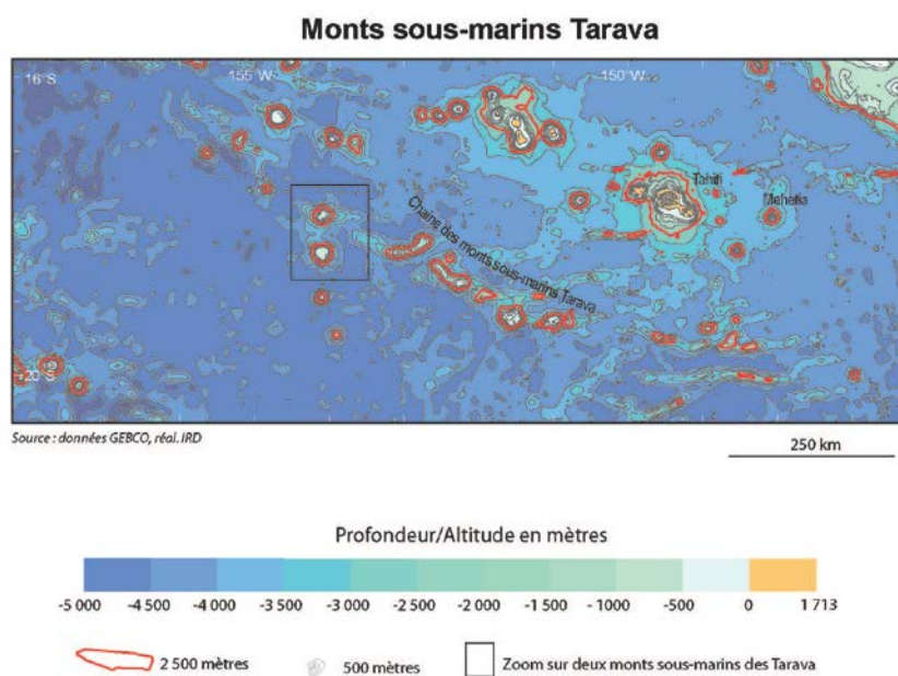
Figure 6 – Bathymétrie de la région des monts Tarava et îles de la Société
