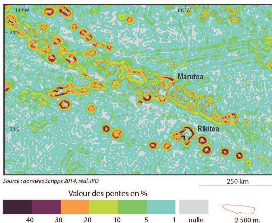
Figure 30 – Carte des pentes de la région des Gambier
