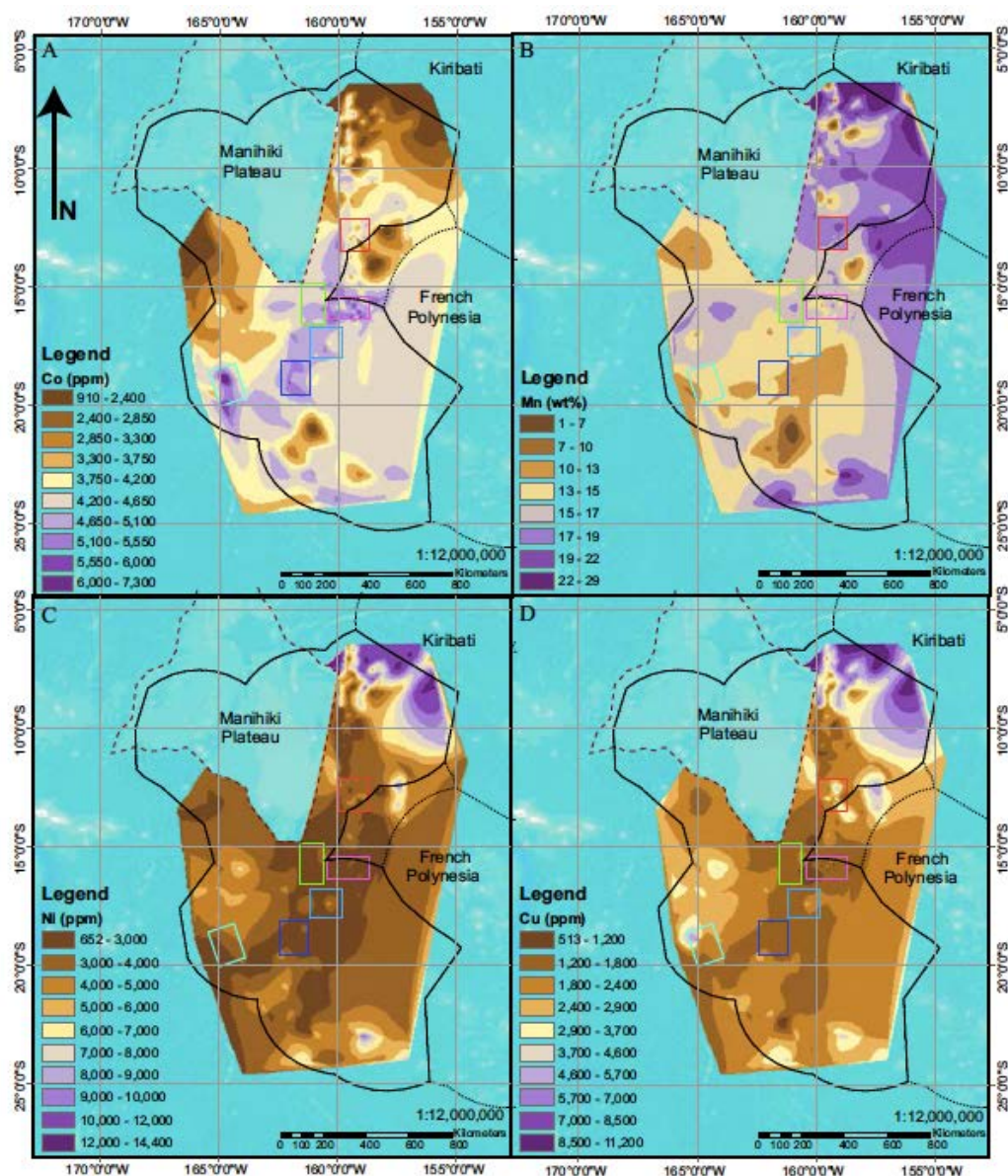
Figure 16 – Concentrations de métaux dans des nodules polymétalliques dans les régions à l'ouest de la ZEE de Polynésie française (Hein et al. , 2015)
