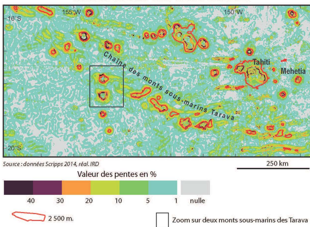
Figure 27 – Carte des pentes de la région des monts sous-marins Tarava et des îles de la Société
