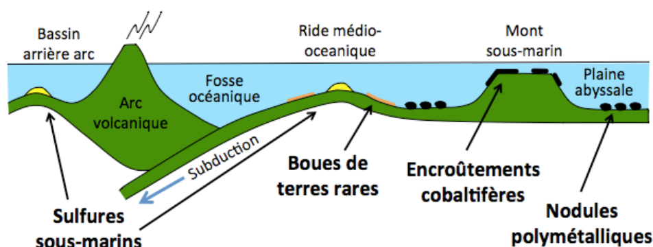
Figure 2 – Schéma montrant le contexte tectonique et l'origine des principaux types de ressources marines
