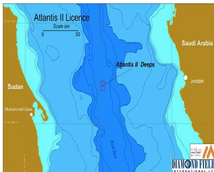
Figure 5 — Localisation pu permis pour le projet Atlantis II (Source : site web de Diamond fields 2 )
