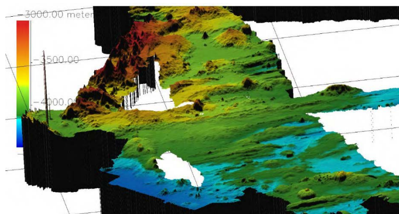
Figure 6 Vue 3D au large des Tuamotu, de 3 000 à plus de 4 000 mètres de profondeur. Source : Ifremer 1 . Crédit image : Ifremer
