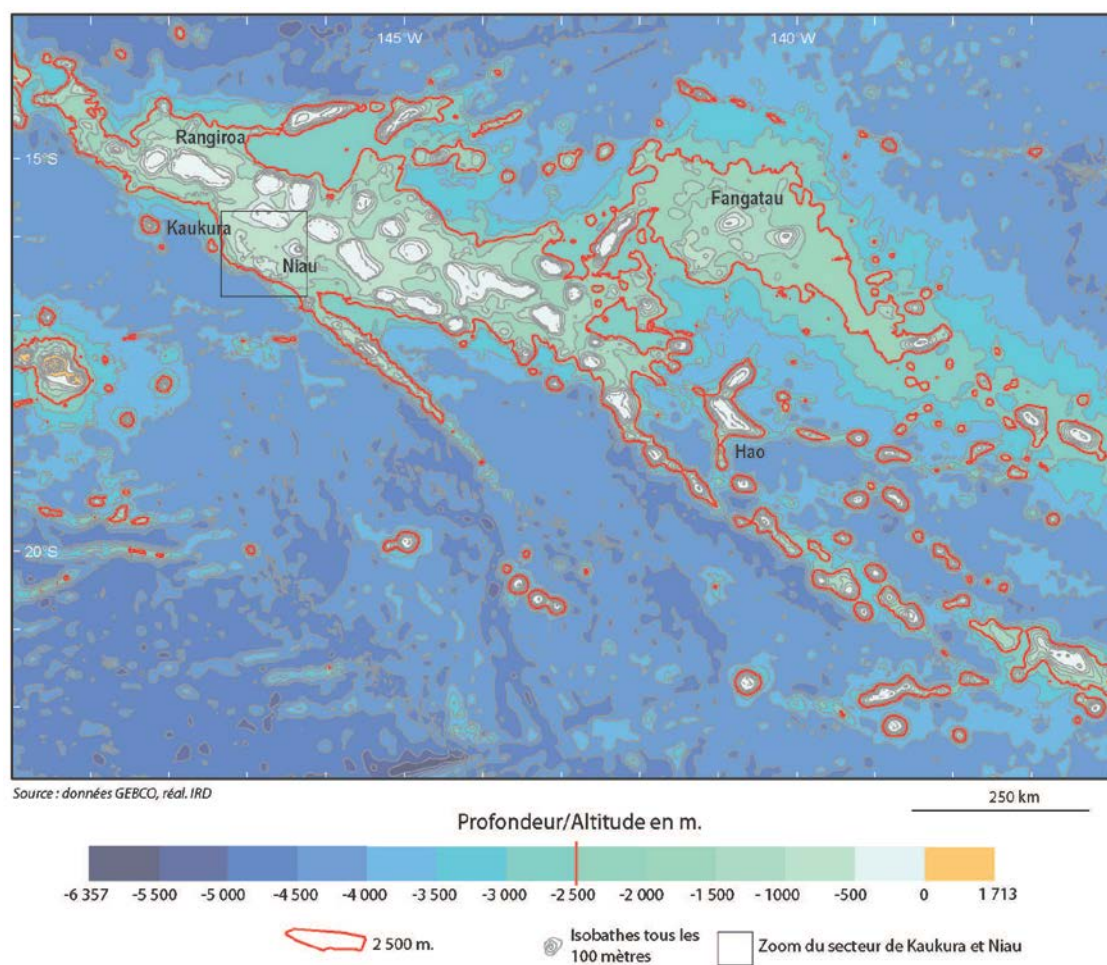
Figure 19 – Bathymétrie de la région des Tuamotu
