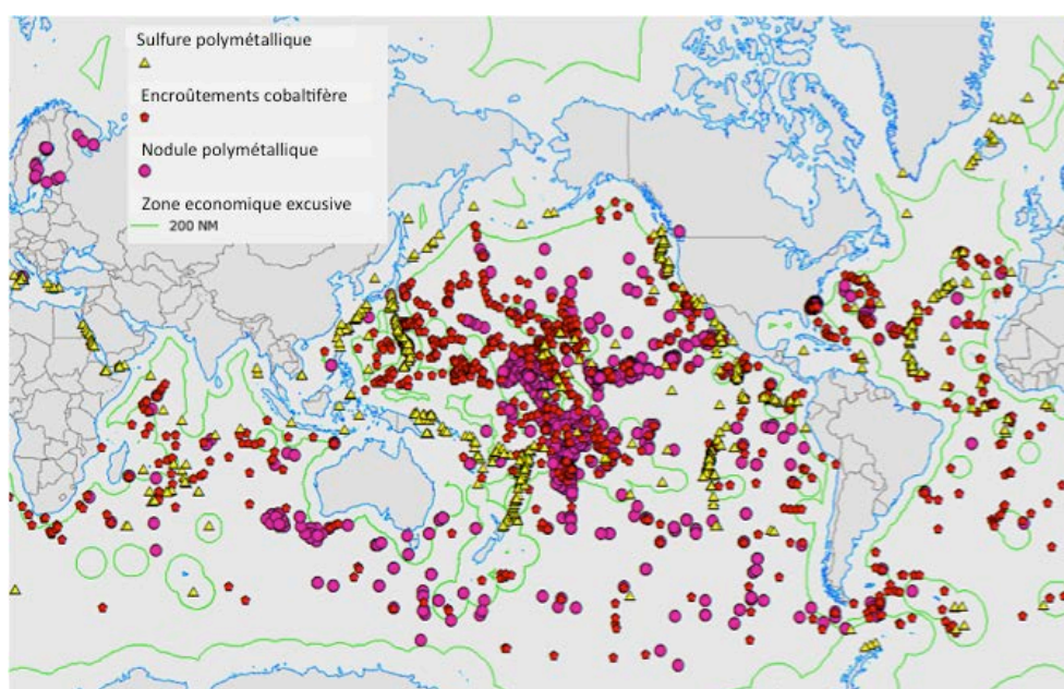
Figure 1 – Distribution globale des trois grands types de ressource minérale marine (ISA, 2014a)
