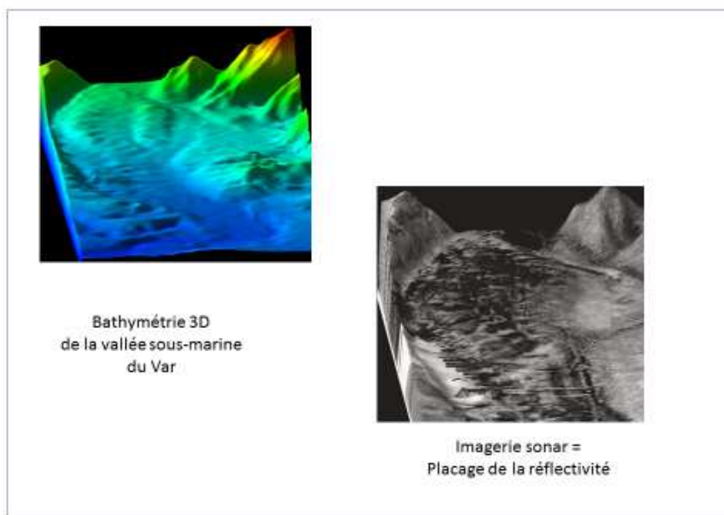
Figure 2 – Exemple de la vallée sous-marine du Var. Les fortes réflectivités traduisent la présence de galets dans le fond de la vallée. © Ifremer B. Savoye
