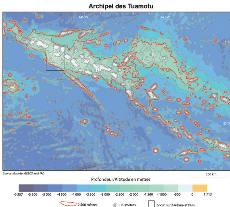
Figure 3 – Bathymétrie de la région de l'archipel des Tuamotu, montrant la répartition des zones où la profondeur est inférieure à 2500 m (isobathe 2500 m en rouge)
