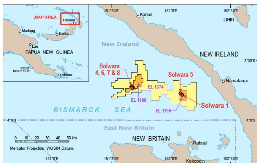
Figure 2 — Zones d'exploration des sulfures sous-marins du groupe Nautilus Minerals
