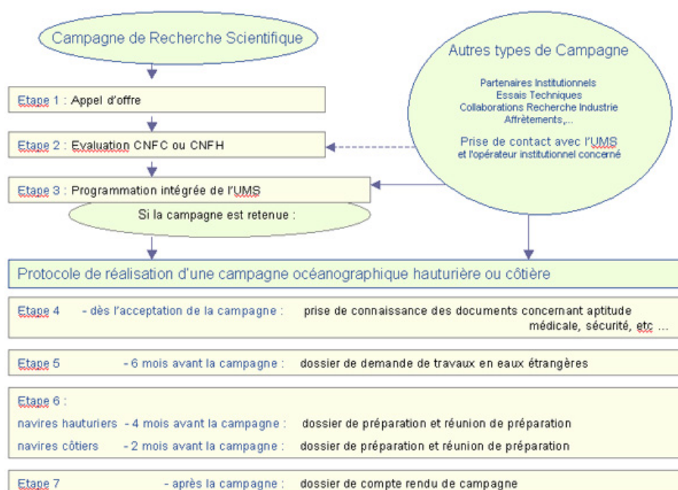
Figure 1 – Processus suivi pour la réalisation d'une campagne océanographique hauturière (Source : http://www.flotteoceanographique.fr/Campagnes-scientifiques/Campagnes-hauturieres )
