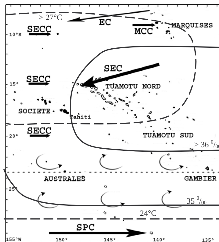
Carte 2 – Courants de surface en Polynésie française : Courant Equatorial (EC), Courant Equatorial Sud (SEC), Contre-Courant Equatorial Sud (SECC), Contre-Courant des Marquises (MCC), Courant du Pacifique Sud (SPC). Les isothermes et isohalines du champ moyen de la température et de la salinité de surface sont respectivement indiqués par des lignes en pointillées et continues (Martinez E., 2006).
