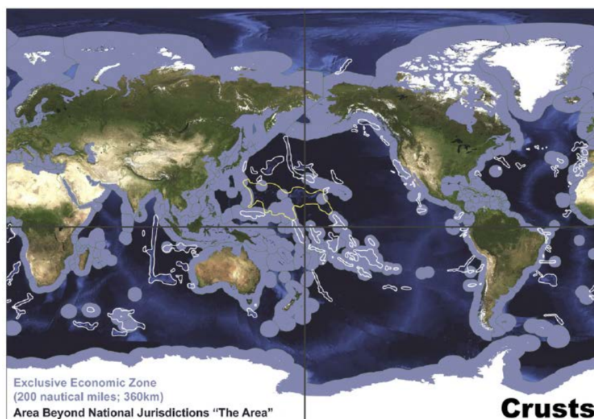
Figure 4 – Distribution d’encroûtements cobaltifères (« zone privilégiée » délimitée en jaune) (Source : Hein et al. 2013)
