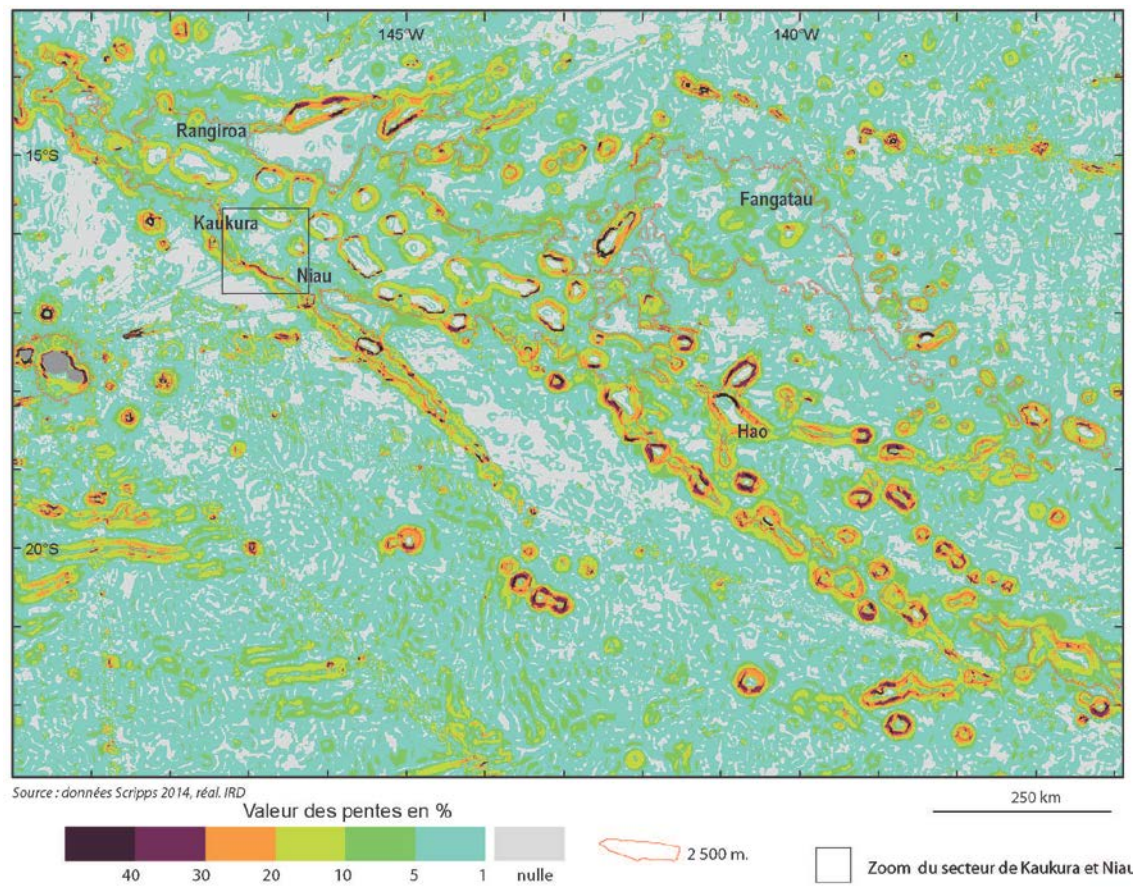
Figure 25 – Carte des pentes de la région des Tuamotu
