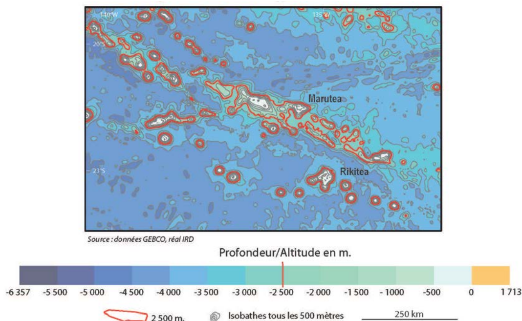
Figure 24 – Bathymétrie de la région des Gambier
