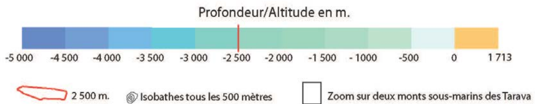
Figure 21 – Bathymétrie de la région des monts sous-marins Tarava et des îles de la Société
