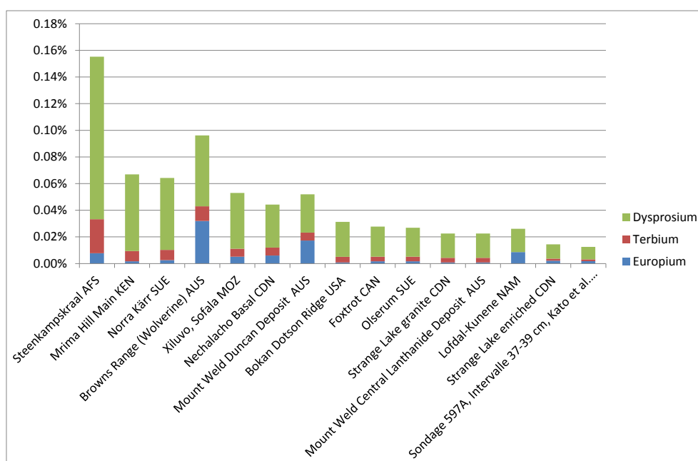
Figure 1 – Comparaison de la teneur en dysprosium, europium et terbium (les 3 terres rares les plus chères, les plus recherchées) dans la meilleure passe minéralisée observée par Kato et al. (2011) parmi 78 forages réalisés dans les boues sédimentaires abyssales du Pacifique, avec les gisements terrestres à teneurs supérieures.
