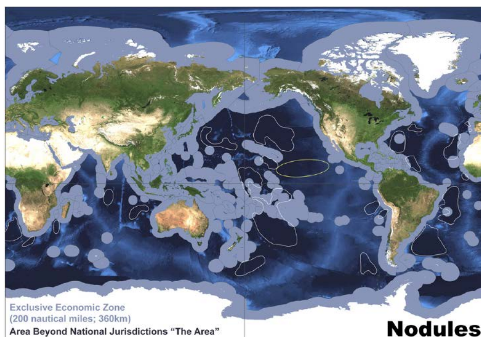
Figure 7 – Distribution des nodules polymétalliques (de Hein et al. 2013)
