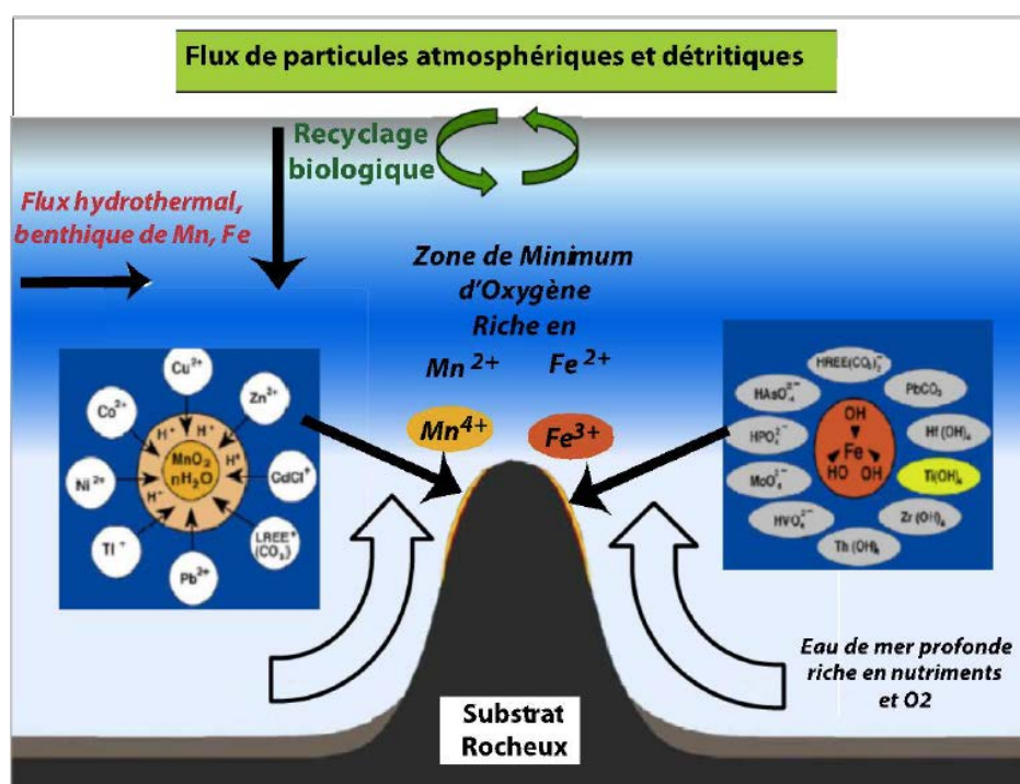
Figure 5 – Modèle de formation des encroûtements cobaltifères (Source : ESCo rapport 2014)
