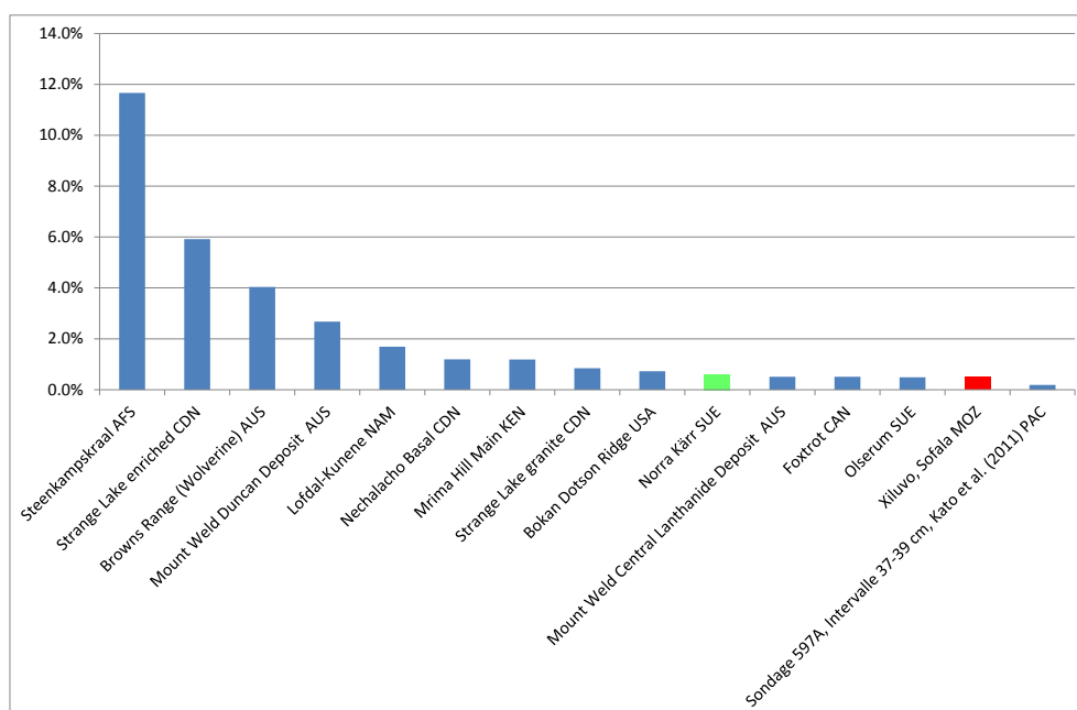
Figure 2 – Comparaison des teneurs totales en terres rares de la meilleure passe de Kato et al. (2011) avec les teneurs totales en terres rares des gisements de la figure 1.
