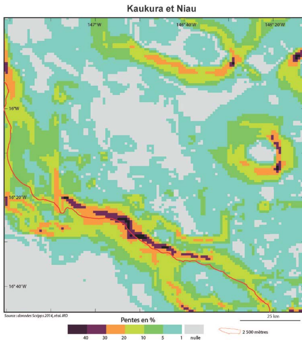
Figure 5 – Carte des pentes de la région de Kaukura et Niau, dans l'archipel des Tuamotu
