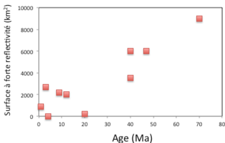
Figure 3 – Corrélation entre âges des édifices volcaniques et superficie de zone de forte réflectivité. Données de Bonneville 2002 ; valeurs maximales pour surfaces réfléchives.
