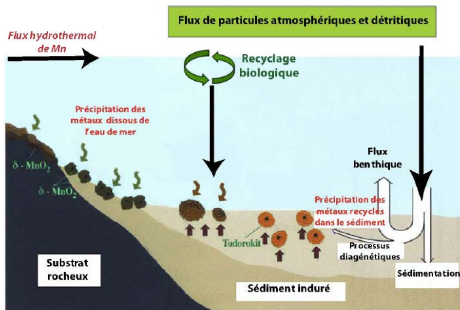
Figure 6 – Modèle de formation des nodules polymétalliques (Source : rapport ESCO Dymont et al., 2014)
