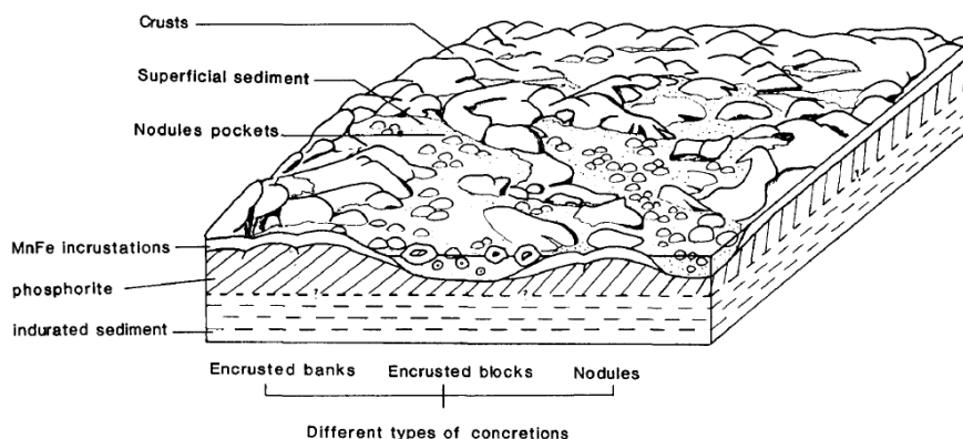
Figure 14 – Dessin de Pichocki et Hoffert (1987) de la surface du plancher océanique de la zone Kaukura.
