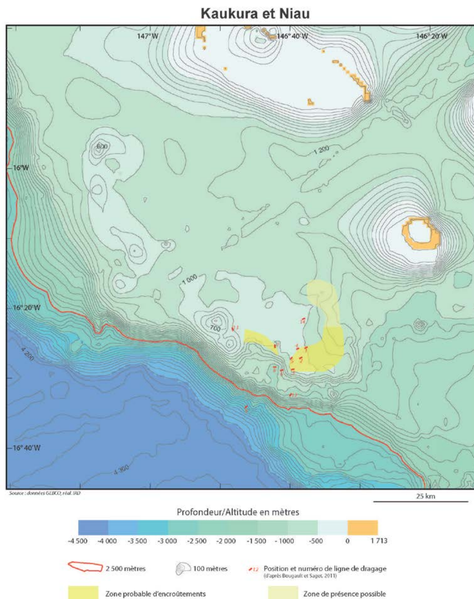
Figure 4 – Bathymétrie de la région de Kaukura et Niau, dans l'archipel des Tuamotu, avec positionnement des prélèvements effectués, d'après Bougault et Saget, 2011.
