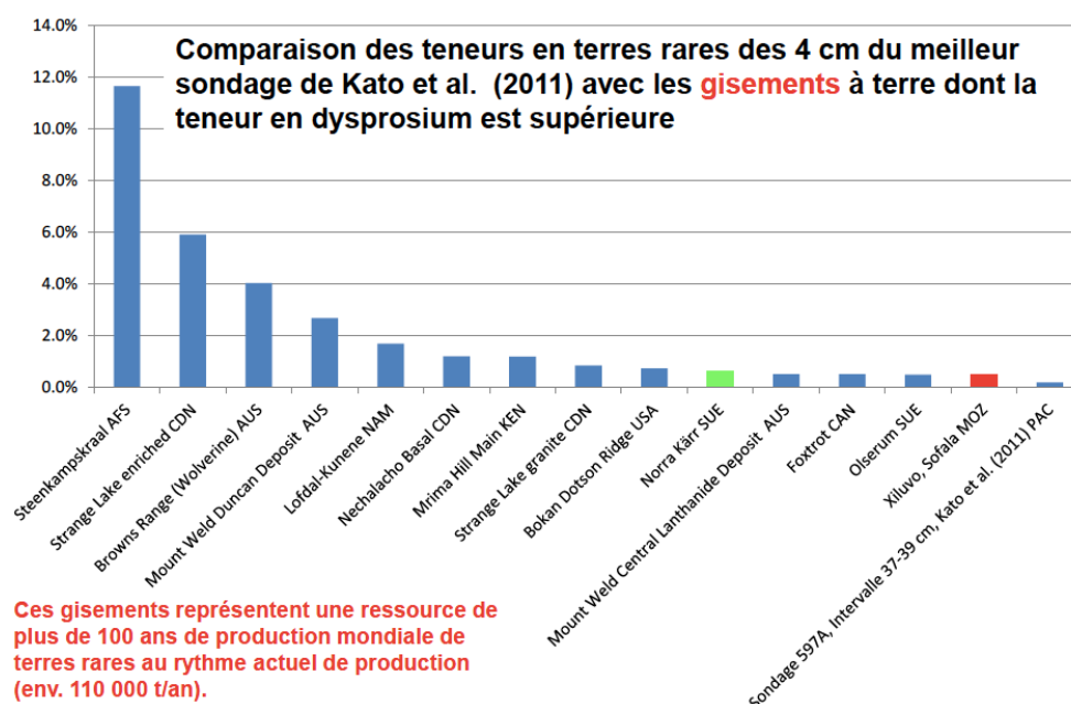
Figure 11 – Les teneurs et les tonnages probables de gisements de terres rares (© BRGM/ P. Christmann - source des données : Kato et al. (2011))
