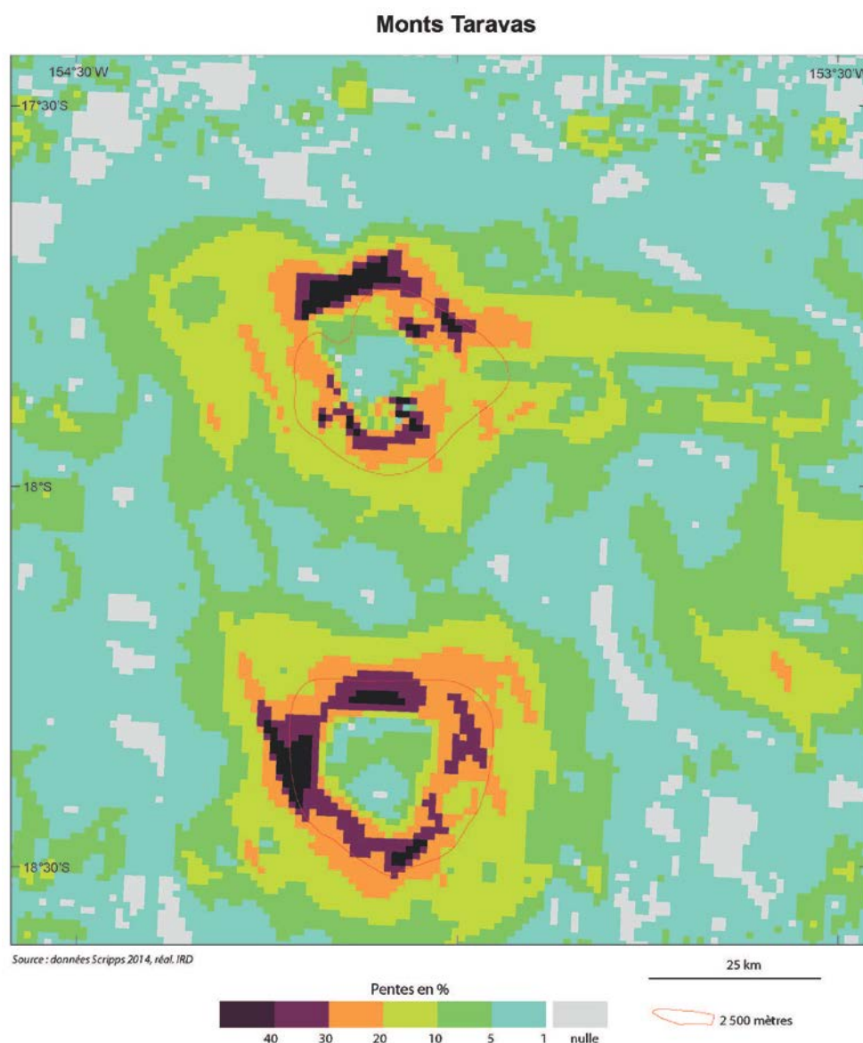
Figure 9 – Carte des pentes de deux monts sous-marins Tarava
