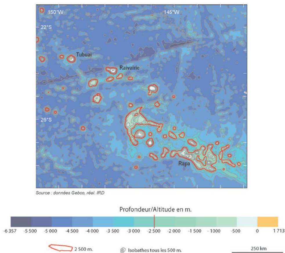
Figure 23 – Bathymétrie de la région des Australes
