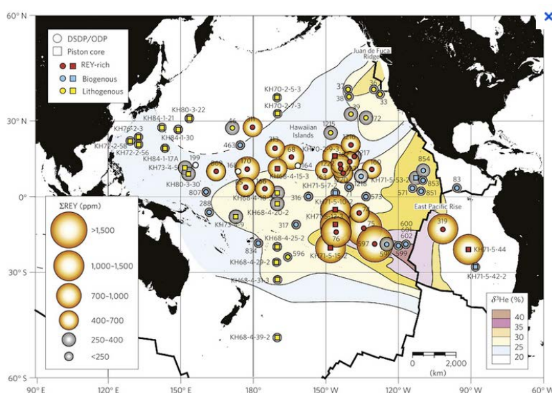
Figure 10 – Carte des prélèvements effectués par Kato et al. (2011)
