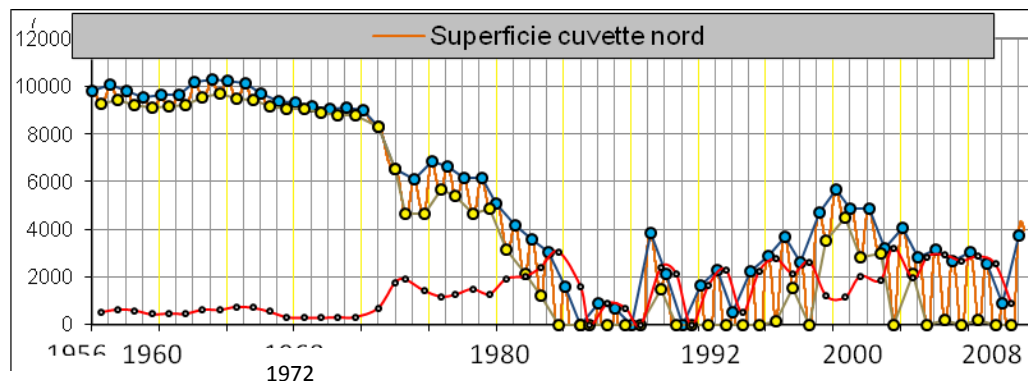
Figure 3 – Évolution des surfaces de marnage en km 2 dans la cuvette nord depuis 1956 ; la représentation de la période 1973-82 est approximative.
