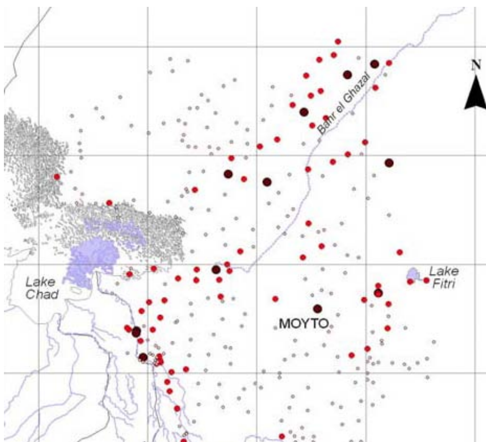
Figure 2 – Les concentrations en fluor dans les eaux souterraines de la partie tchadienne du bassin Points clairs, concentration inférieure à 0,5 mg/L ; rouge entre 0,5 et 1,5 ; noir au dessus de 1,5 mg/L et jusqu'à 3,3 mg/L (d'après CBLT-BGR, 2010).
