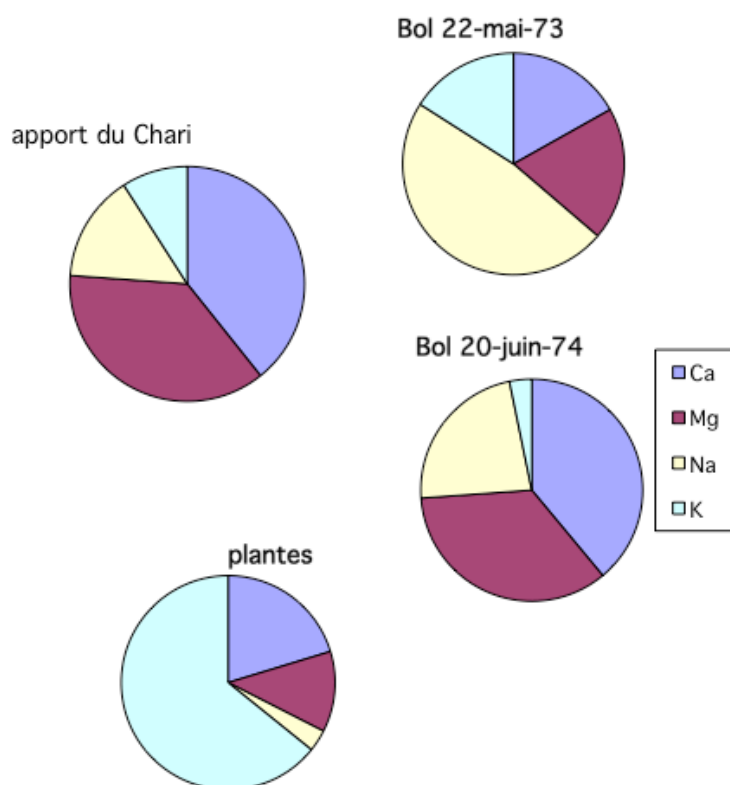
Figure 1 – Composition en ions majeurs (mg/L) de l'apport moyen du Chari, de l'eau du Lac en phase de Moyen Tchad (exemple de Bol, 22 mai 1973, conductivité 400 microSiemens) et en phase de Petit Tchad (Bol, 20 juin 1974, conductivité 400 microSiemens) en présence d'une forte densité de plantes aquatiques dont la composition est indiquée dans le graphique plantes (données Lemoalle).
