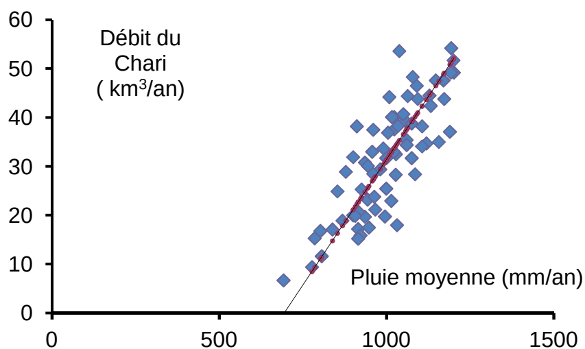
Figure 5 – Relation entre la pluie sur le bassin du Chari-Logone et le débit du fleuve. Pour une variation de 10 % de la pluie, le débit annuel du fleuve varie de 30 %.
