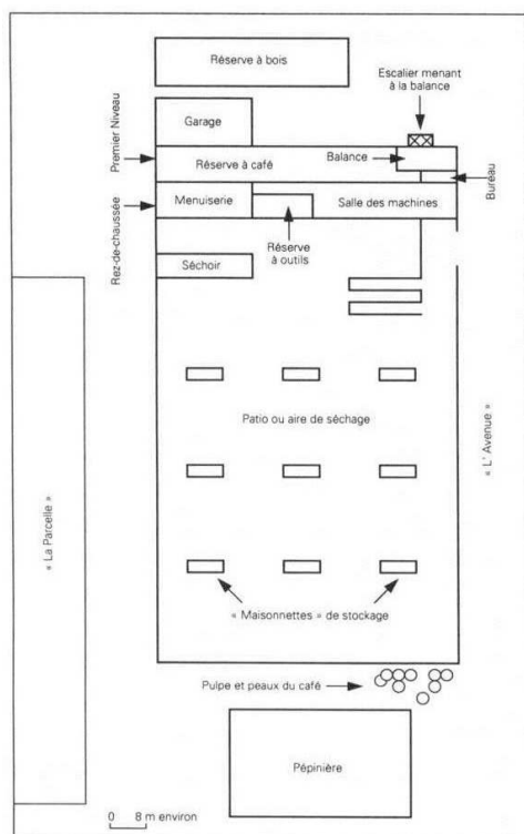
Figure 7. Plan du beneficio.
