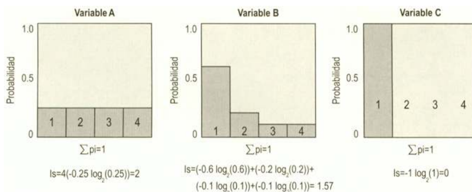
Figura 38: Cálculo del índice de Shannon y la medida de la entropía. Tres casos de distribución de la frecuencia y el cálculo del índice de Shannon
