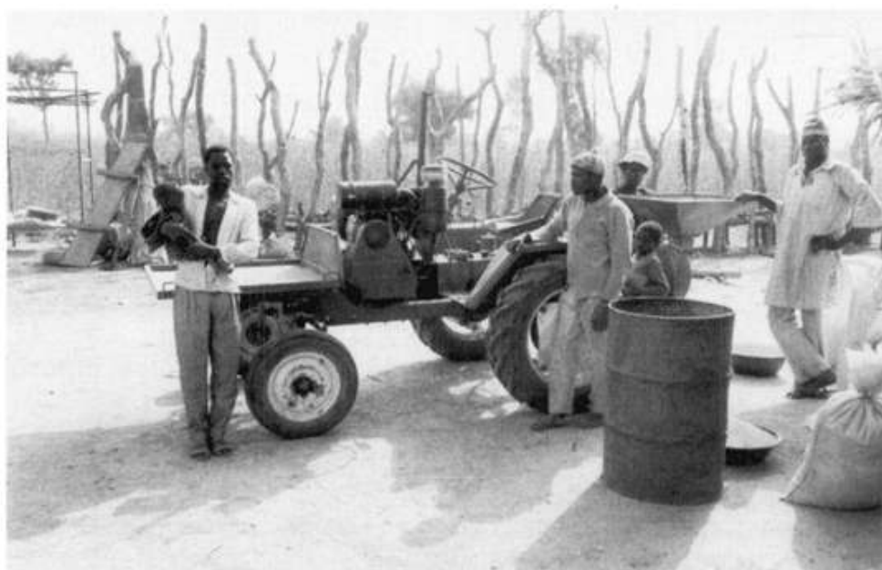
11. Le tracteur « Bouyer » de 30 chevaux, monté dans les ateliers d'assemblage de la Sofitex de Bobo-Dioulasso. Une prise de force à l'arrière lui permet d'entraîner un moulin à céréales ou une égreneuse à maïs. Une charge de 500 kg peut être transportée sur le petit plateau à l'avant du tracteur.
