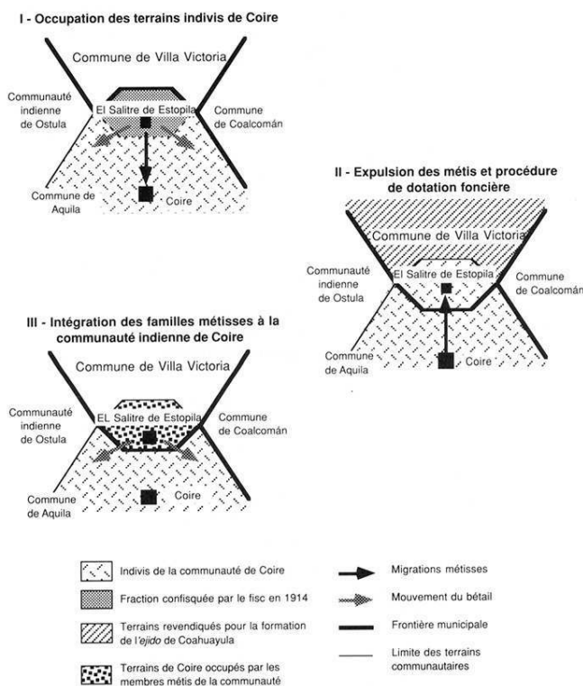
Figure 22. Représentation simplifiée des conflits fonciers entre la communauté indienne de Coire et le hameau métis de El Salitre de Estopila.
