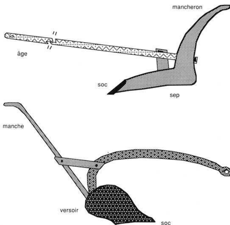
Figure 17. Araire et charrue utilisés dans la Sierra de Coalcomán.
