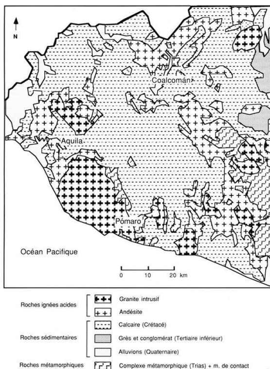
Figure 12. Carte géologique de la Sierra Madre del Sur (État du Michoacán).
